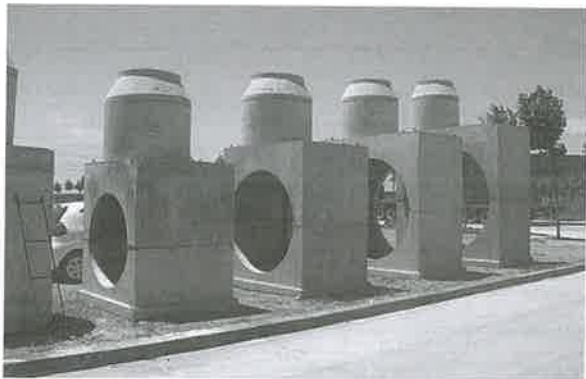
图3: 装配式预制砼(节) (矩形检查井)
